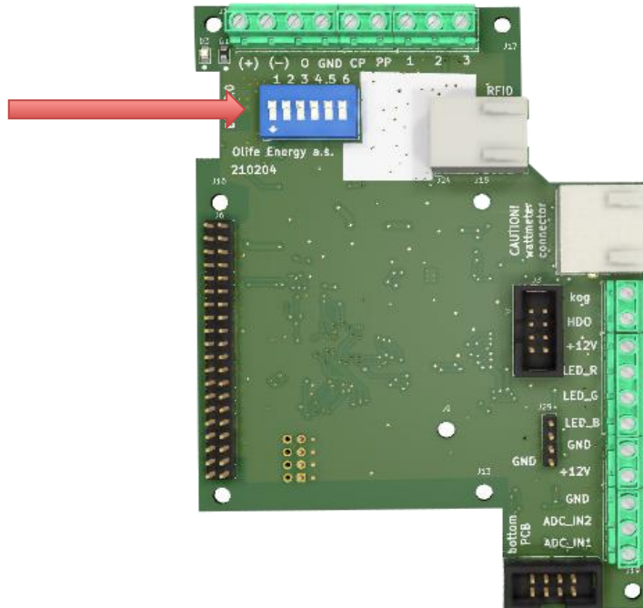
Obrázek 11: Vyznačení DIP-switchu na řídicí desce wallboxu
