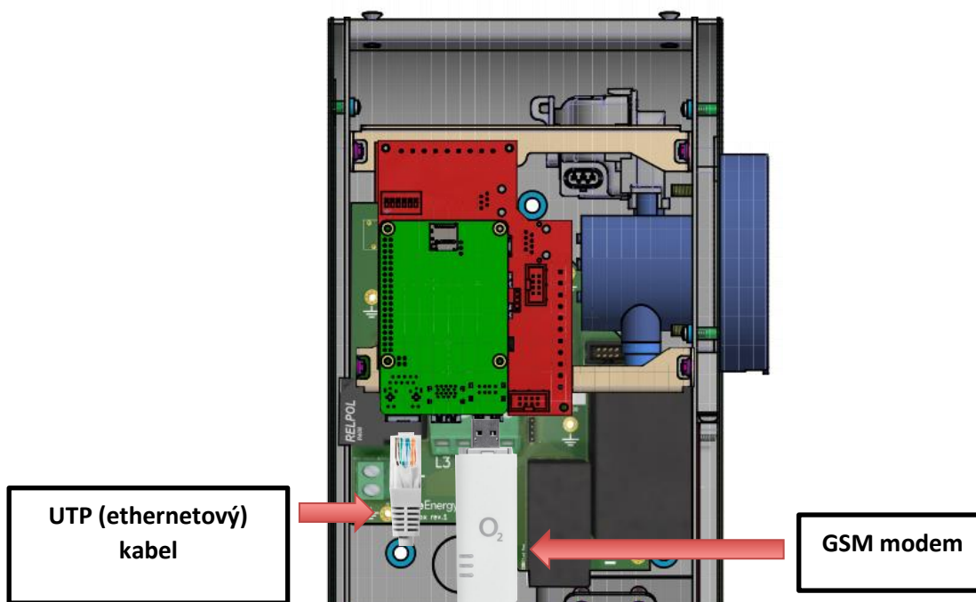
Obrázek 10: Zapojení GSM modemu/síťového kabelu
