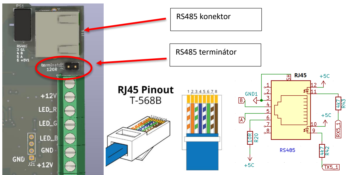
Obrázek 15: RS485 zapojení
